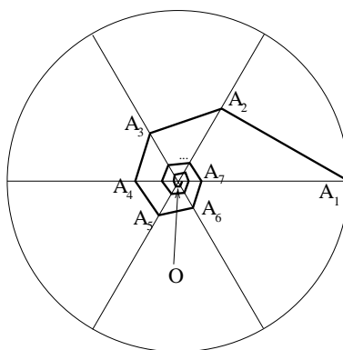
FIG. 1: construction d'une spirale
